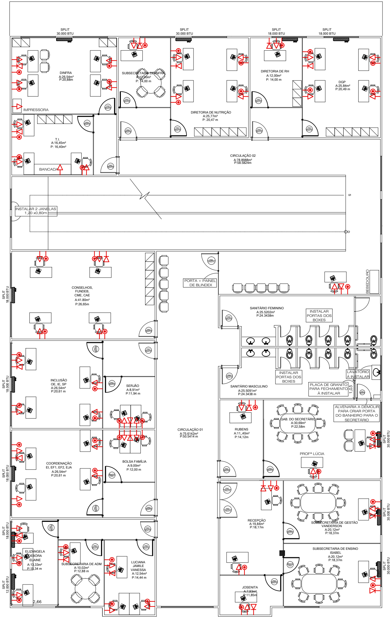
PLANTA BAIXA - 2º PAV. - ADEQUAÇÃO DO PRÉDIO PARA SEMED LOCAÇÃO DOS PONTOS ELÉTRICOS - SEM ESCALA
