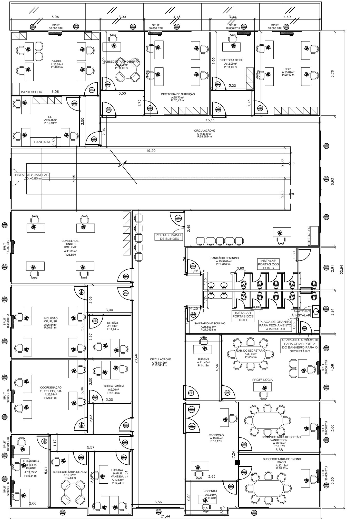
PLANTA BAIXA - 2º PAV. - ADEQUAÇÃO DO PRÉDIO PARA SEMED SEM ESCALA
