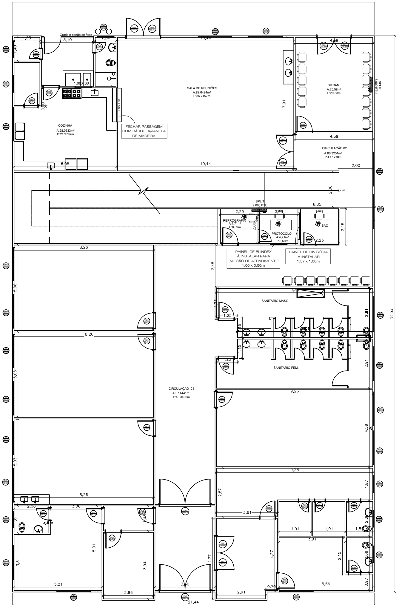
PLANTA BAIXA - 1ºPAV. - ADEQUAÇÃO DO PRÉDIO PARA SEMED
